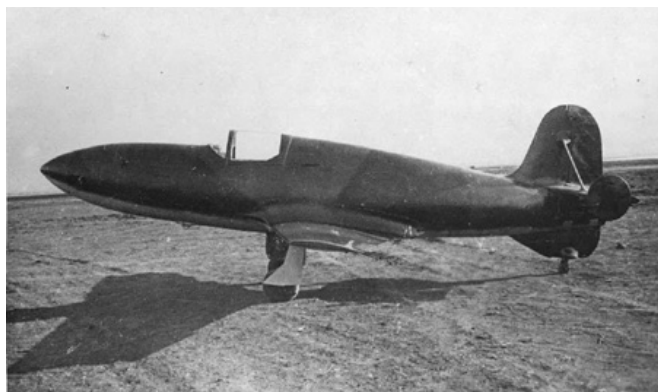
Рис. 1. Самолёт БИ-1 на аэродроме Кольцово (город Свердловск) в мае 1942 года. РГАНТД. Ф. 107, оп.2, д.6 [4]
